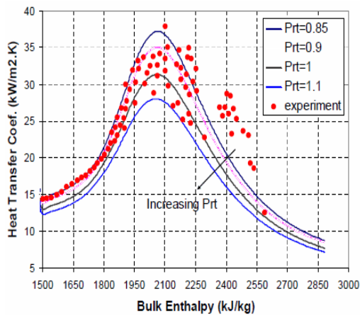
شکل ۹: مقایسه‌ی ضریب انتقال حرارت حاصل از نتایج حل عددی برای اعداد پراتنل ثابت با نتایج تجربی بازرگان و همکاران [۲۷]
