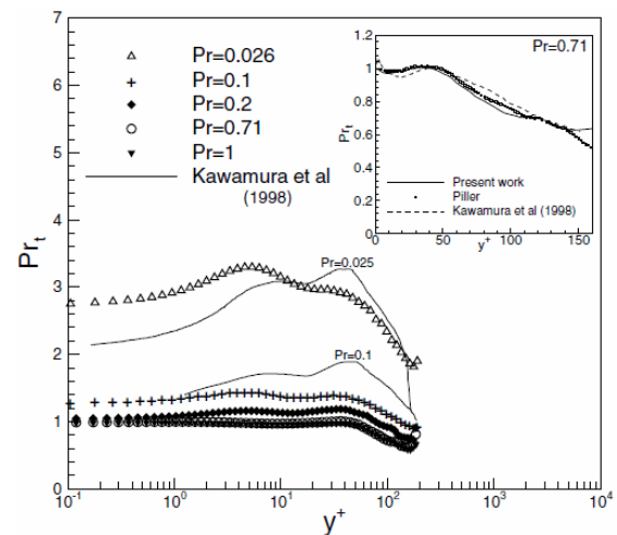
شکل ۱۱: توزیع عدد پرانتل آشفتگی [۲۸]
