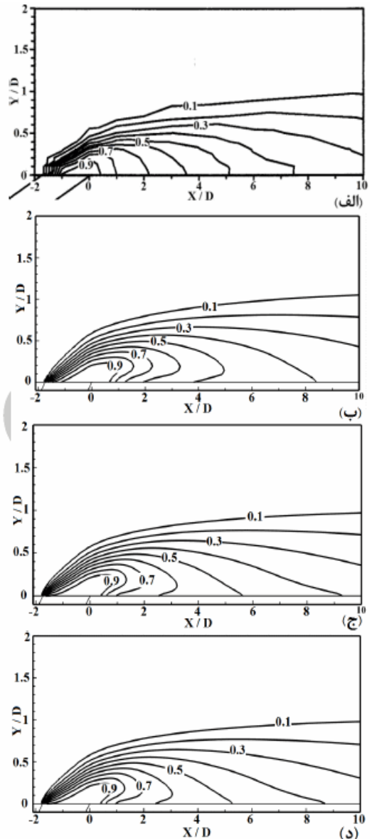
شکل ۸: توزیع دمای بی‌بعد، (الف) مقدار تجربی (ب) پراتنل آشفته ۰/۸۵ (ج) پراتنل آشفته ۰/۷۵ (د) پراتنل آشفته ۰/۷ [۲۴]
