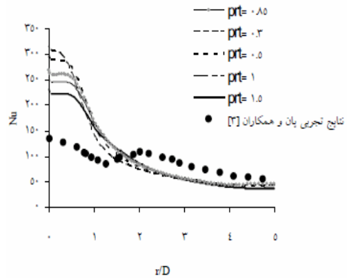
شکل ۵: مقایسه‌ی مدل آشفتگی رینولدز پایین k-\epsilon با اعداد پراتل آشفتگی مختلف با نتایج تجربی (ان L = 2D ) [۲۱]
