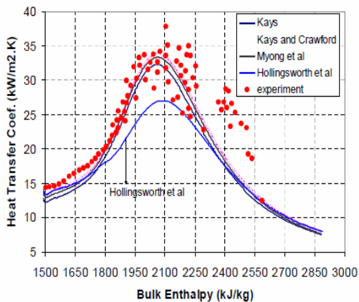
شکل ۱۰: مقایسه‌ی ضریب انتقال حرارت حاصل از نتایج حل عددی برای اعداد پراتنل متغیر با نتایج بازرگان و همکاران [۲۷]
