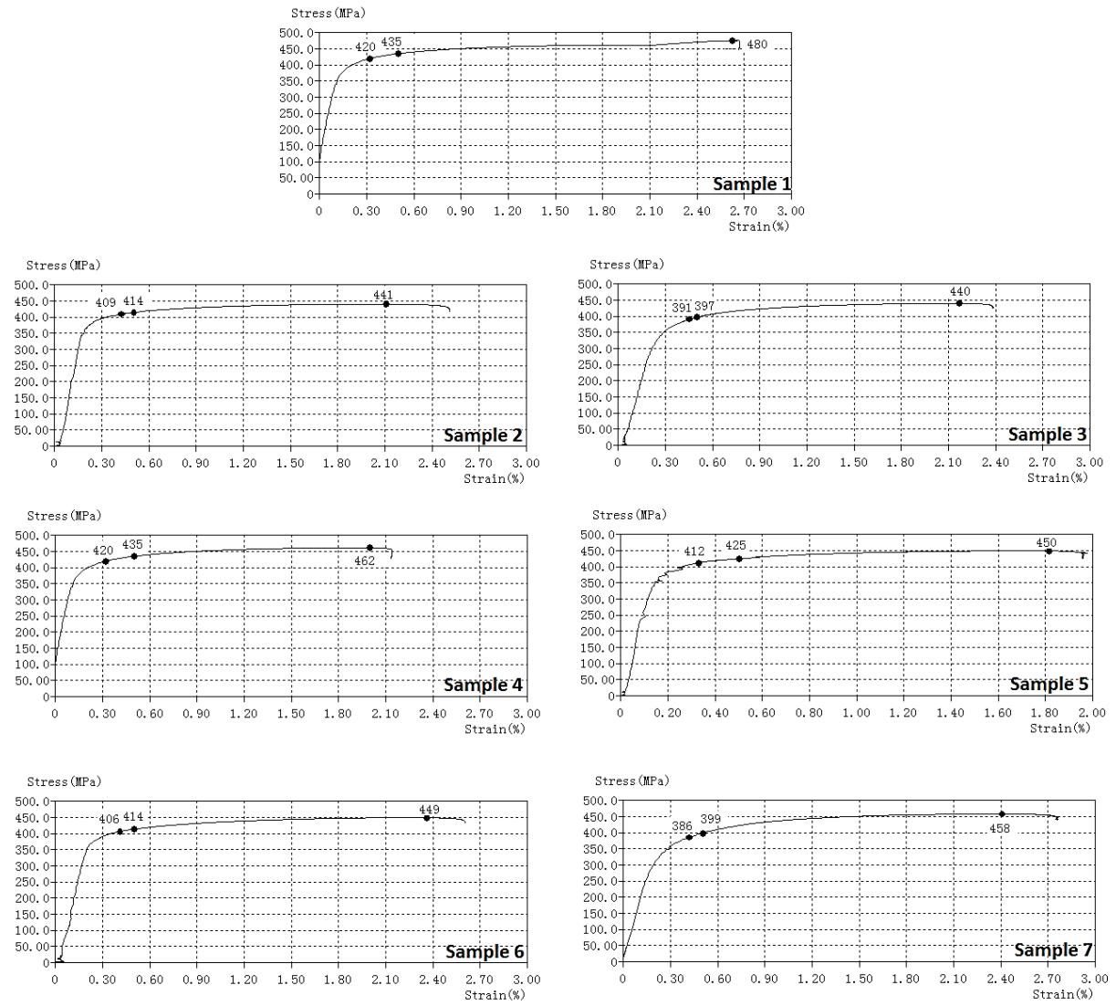
شکل ۶: نمودار تنش- کرنش حاصل از تست کشش نمونه‌های مختلف
