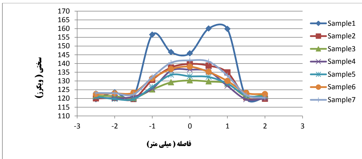
شکل ۷: نمودار تغییرات سختی در نمونه‌های مختلف
