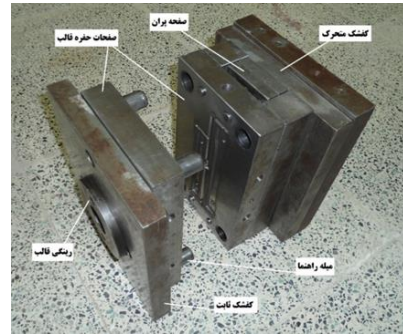
شکل ۴: قالب تزریق
