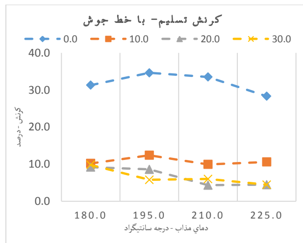
شکل ۱۱: تغییرات کرنش تسلیم بر حسب دمای مذاب در نمونه های با خط جوش
